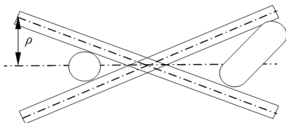
Рис. 6. Схема просіювання зернівки крізь дві соломини, коли соломини перетинаються
