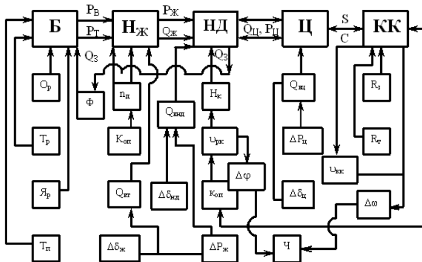
Рис. 1. Діагностична модель гідравлічного привода рульового керування комбайна: Б – бак; НЖ – насос підживлення; НД – насос-дозатор; Ц – гідроциліндри; КК – керовані колеса; Тп – температура повітря; Тр – температура робочої рідини; Ор – рівень робочої рідини в баку; Яр – якість робочої рідини; Ф – фільтр; Qз – злив робочої рідини в бак; Рв, Рт – тиск або вакуум в усмоктувальній магістралі; Qж, Рж – подача і тиск робочої рідини на виході насоса живлення; пд – частота обертання колінчастого вала двигуна; Коп – команда оператора;
