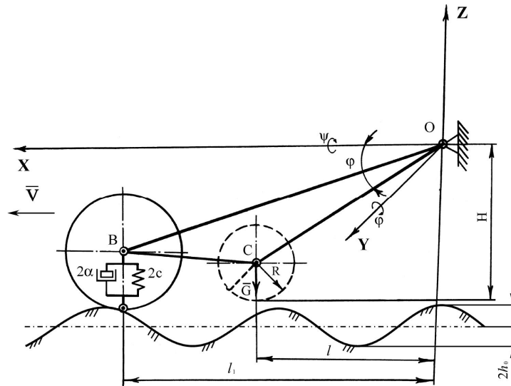
Рис. 1. Еквівалентна схема фронтально навішеної гичкозбиральної машини.
