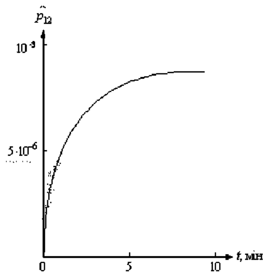
Рис. 2. Залежність вірогідності утворення вільних радикальних пар p_{12} в насінні гороху від часу дії зовнішньої ЕМВ при P = 10 мкВт/см 2 , f = 47,6 ГГц.
