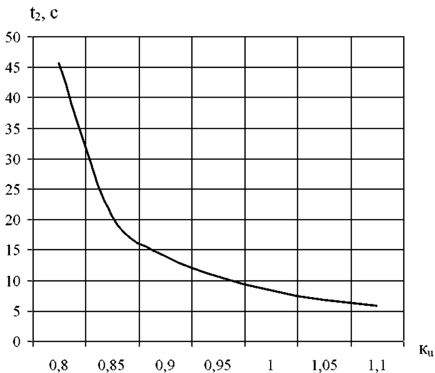
Рис. 4. Зависимость времени разбега электродвигателя на втором участке в функции k_u при \frac{I}{M_n} = 0,05 и k_3 = 1
