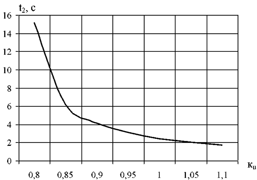
Рис. 6. Зависимость времени разбега электродвигателя на третьем участке в функции k_u при \frac{I}{M_n} = 0,05 и k_3 = 0,9
