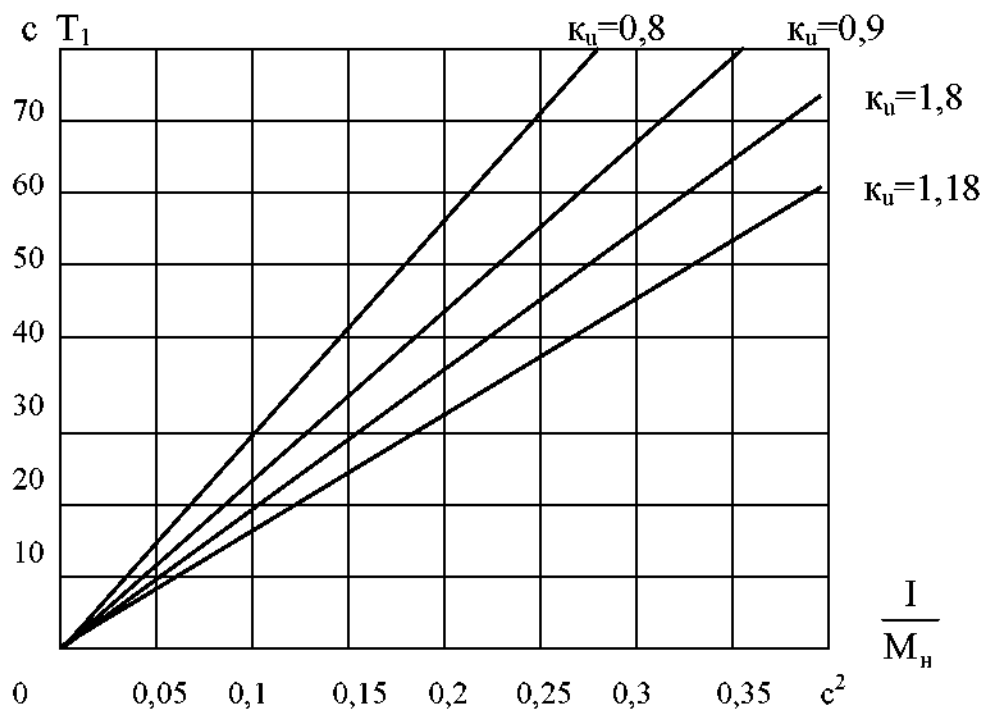
Рис. 3. Зависимость электромеханической постоянной времени T_2 в функции \frac{I}{M_n} при k_3 = 1
