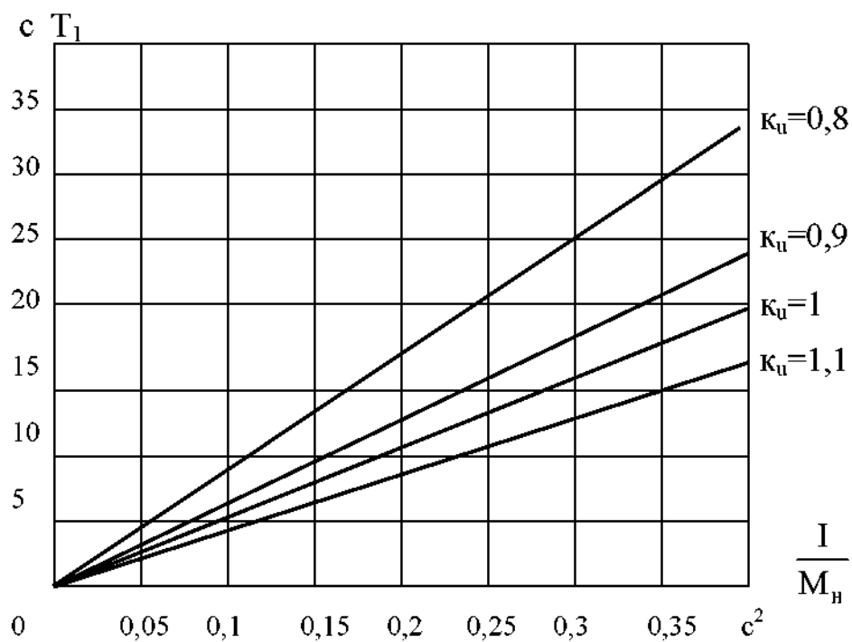
Рис. 5. Зависимость электромеханической постоянной времени T_3 в функции \frac{I}{M_n} при k_3 = 0,9
